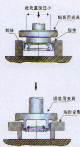
骨架油封不正确的组装
