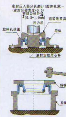
骨架油封的正确组装
