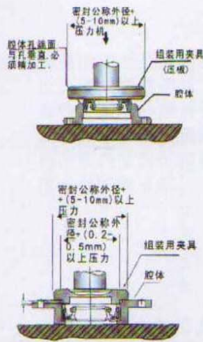
骨架油封的正确组装
